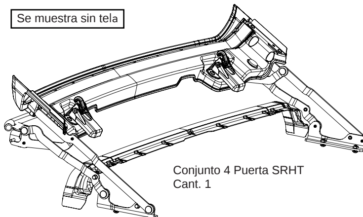
Riel de la puerta: Superior derecho Parte N° 597.34 Cant. 1
